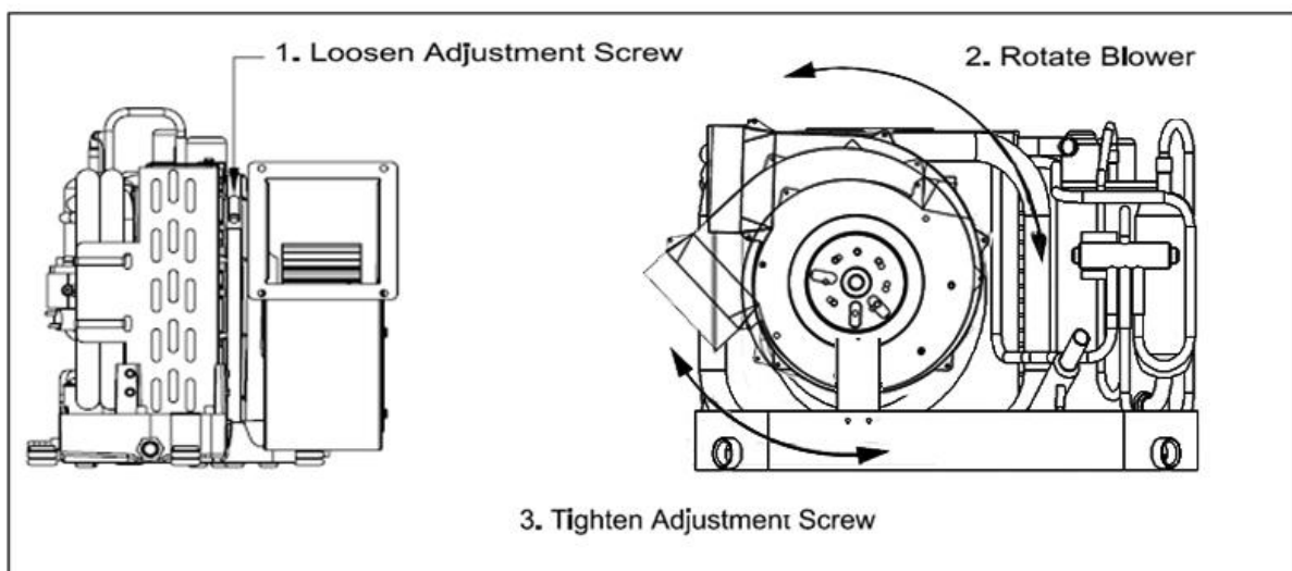
FIGURE 3. Fan motor rotation overview
